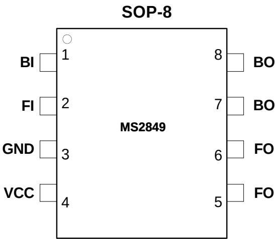
图 1. 顶视图
