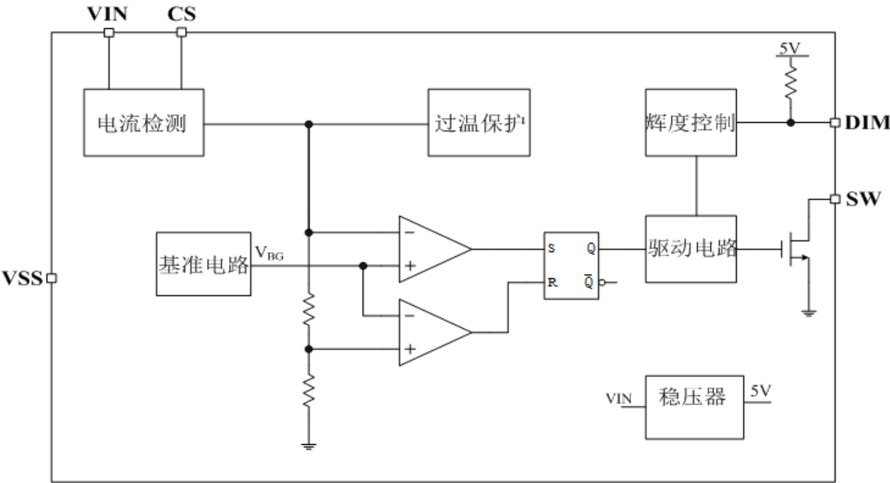
内部电路方框图
