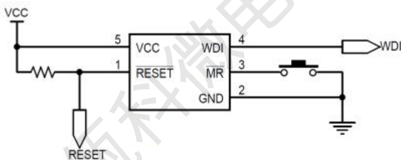
图 1 典型应用图
