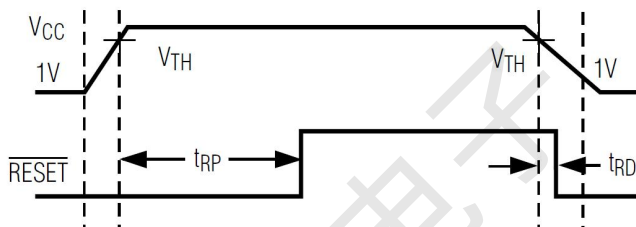
图 4 RESET#时序图
