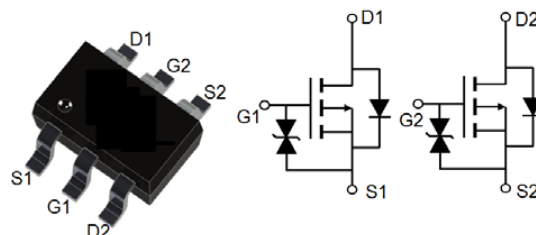
SOT363
