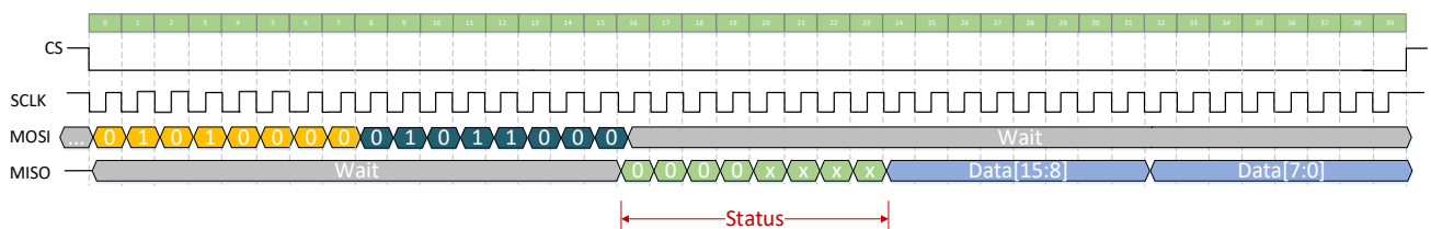
图 15-2. 读寄存器 0x16 SPI 时序图
