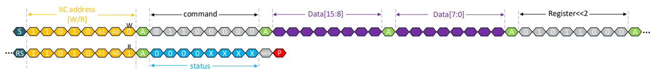
图 15-8. 写寄存器 0x16 I2C 时序图
