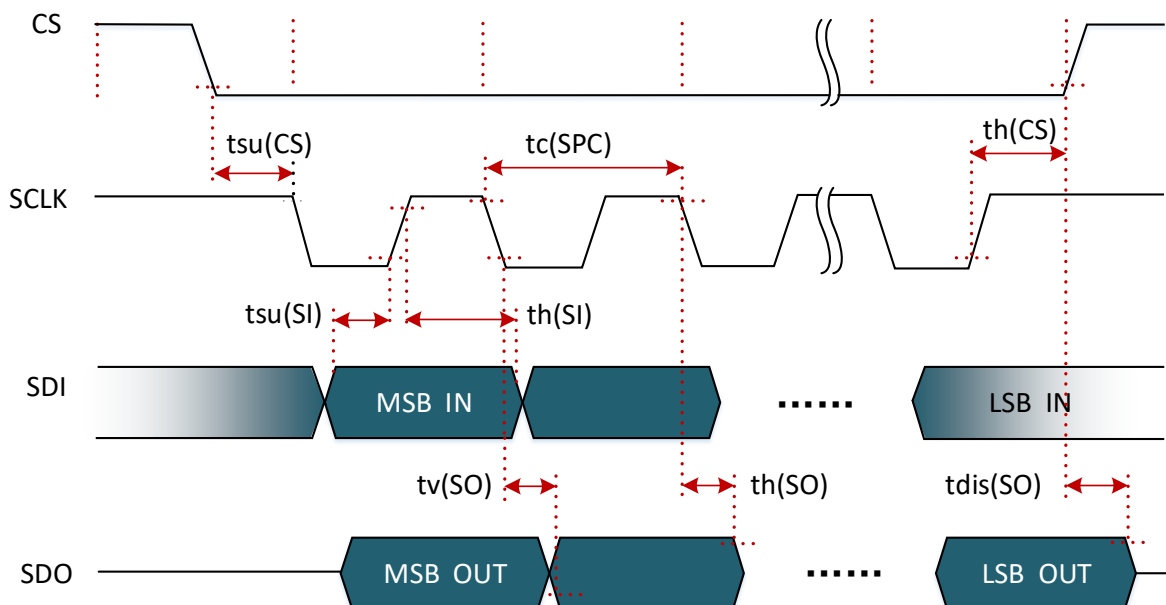
图 12-1 SPI 时序图
