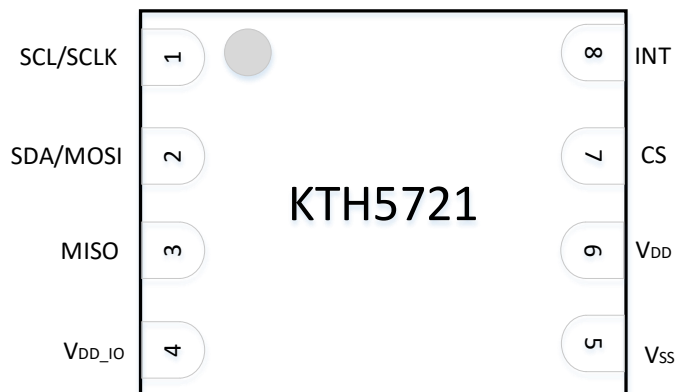
图 5-2. DFN2x2.5 8-Pin 顶视图
