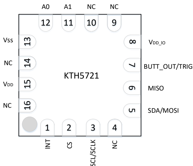
图 5-1.QFN3x3 16-Pin 顶视图
