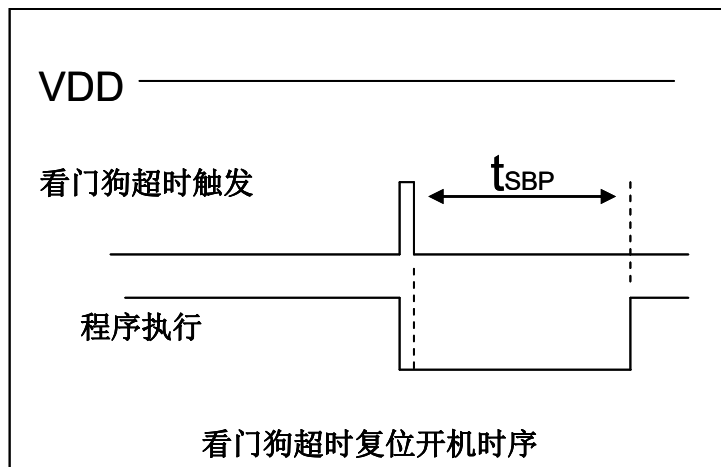
图 11：看门狗定时器超时溢出的相关时序
