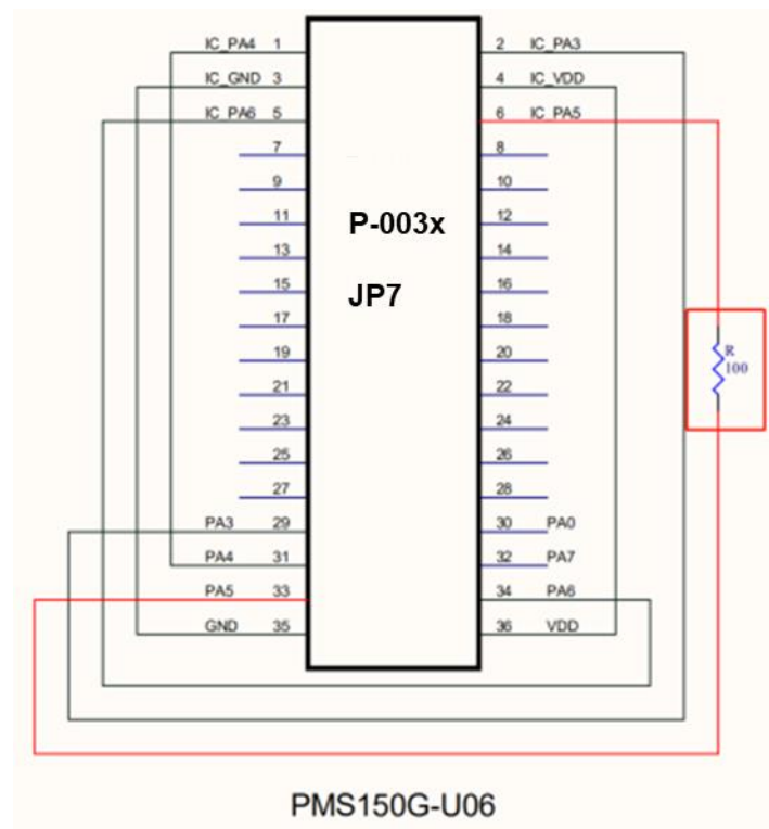
图 16: JP7 连接原理图
