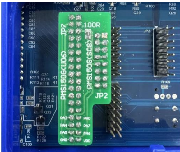
图 14: JP7 连接实物图
