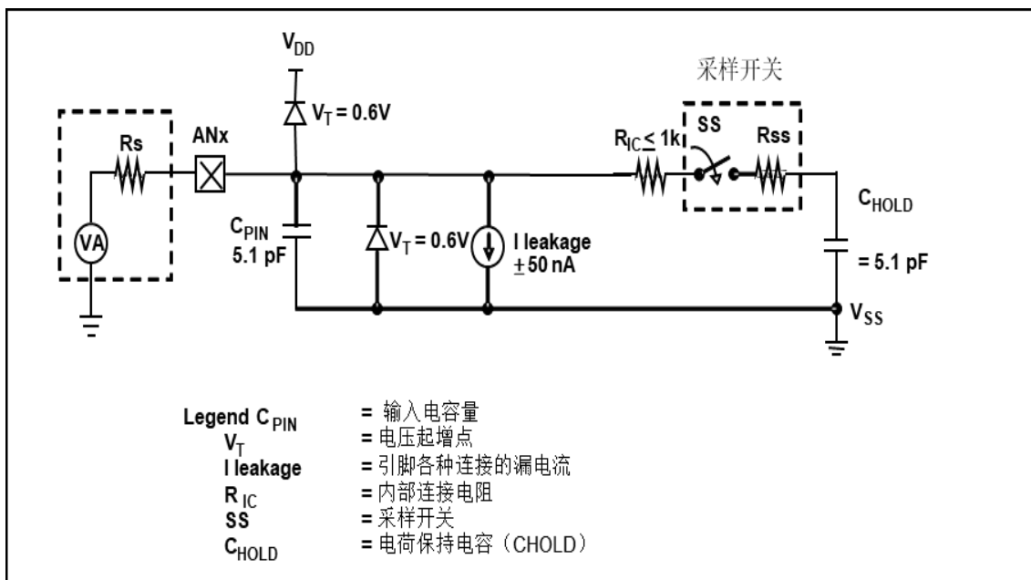
图 20：模拟输入模型
