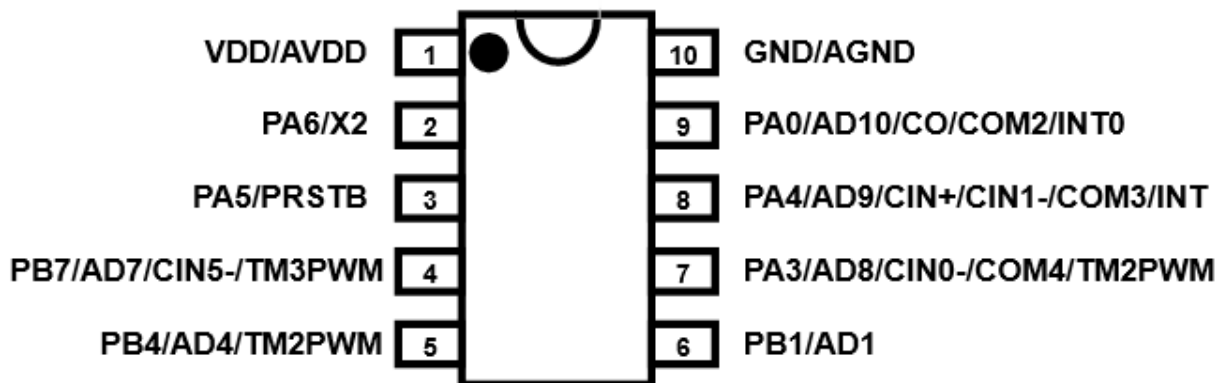
PFS122B-M10 (MSOP10-118mil)
