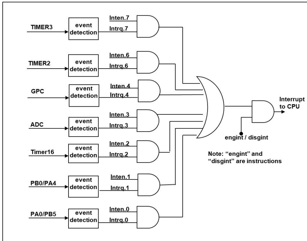
图 17：中断控制器硬件框图
