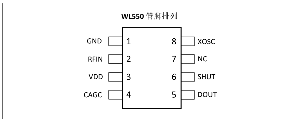
图 2 WL550 管脚排列图
