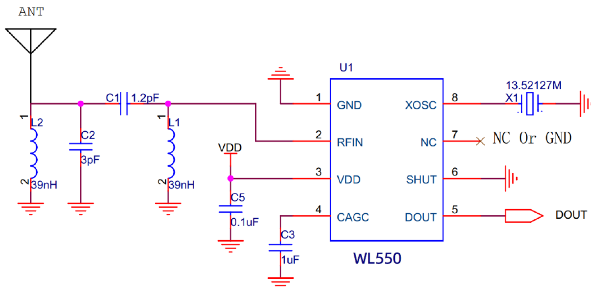
图 3 WL550-433M 典型应用原理图
