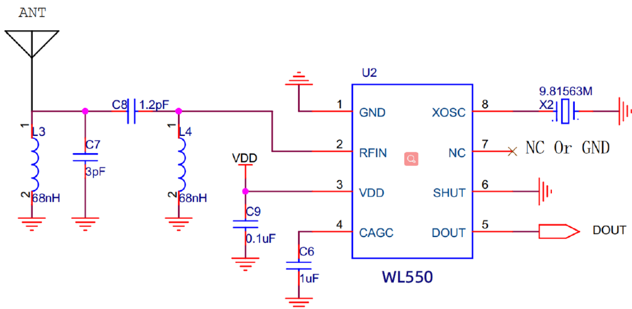
图 4 WL550-315M 典型应用原理图
