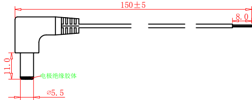
电源连接线
