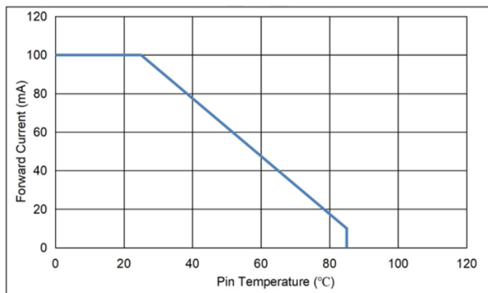
Fig 4 Pin Temperature Vs Forward Current 引脚温度与正向电流特性曲线
