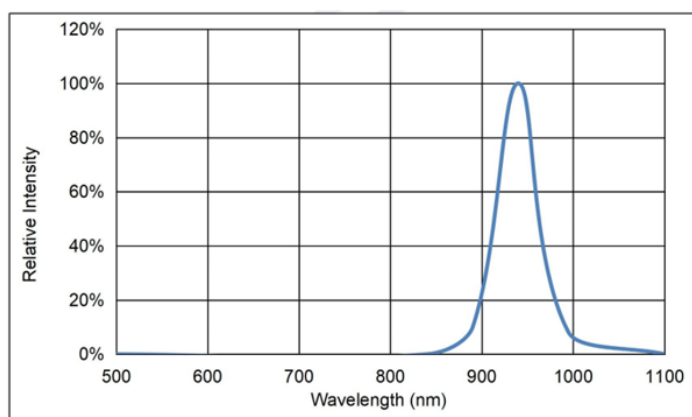
Fig 5 Spectrum Distribution 光谱分布特性曲线
