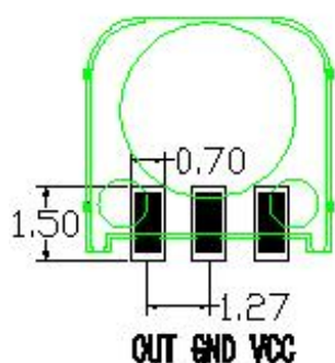
正贴建议焊盘分布
