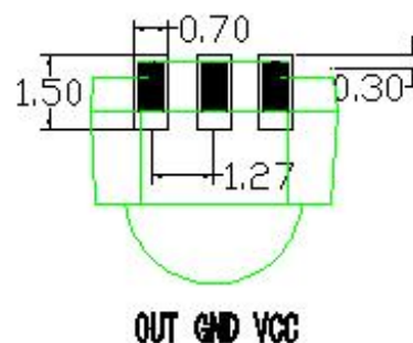
侧贴建议焊盘分布
