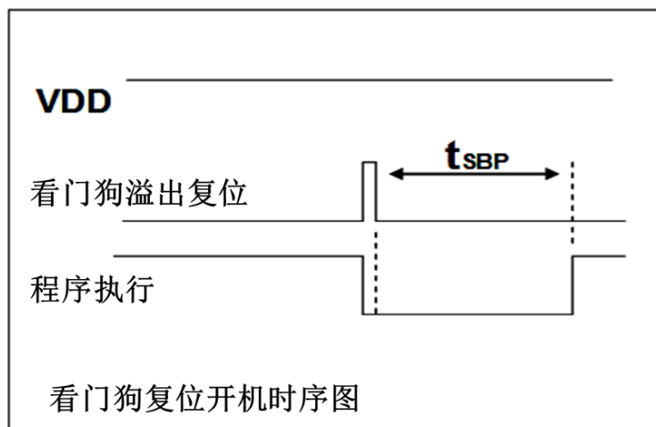
图 18：看门狗超时溢出时序图
