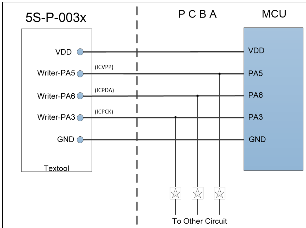
图 24：在板烧录示意图
