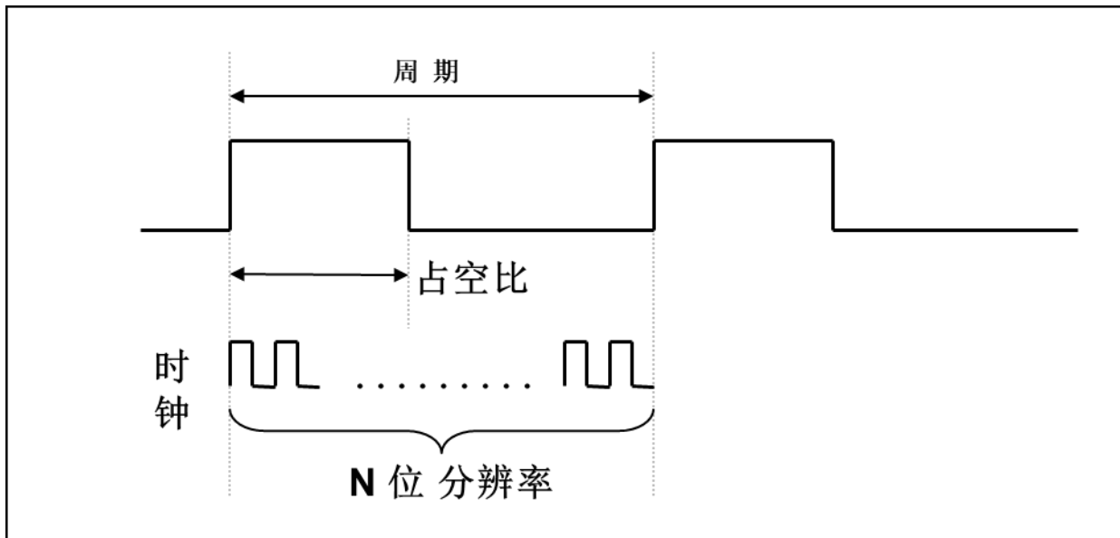
图 14: PWM 输出波形
