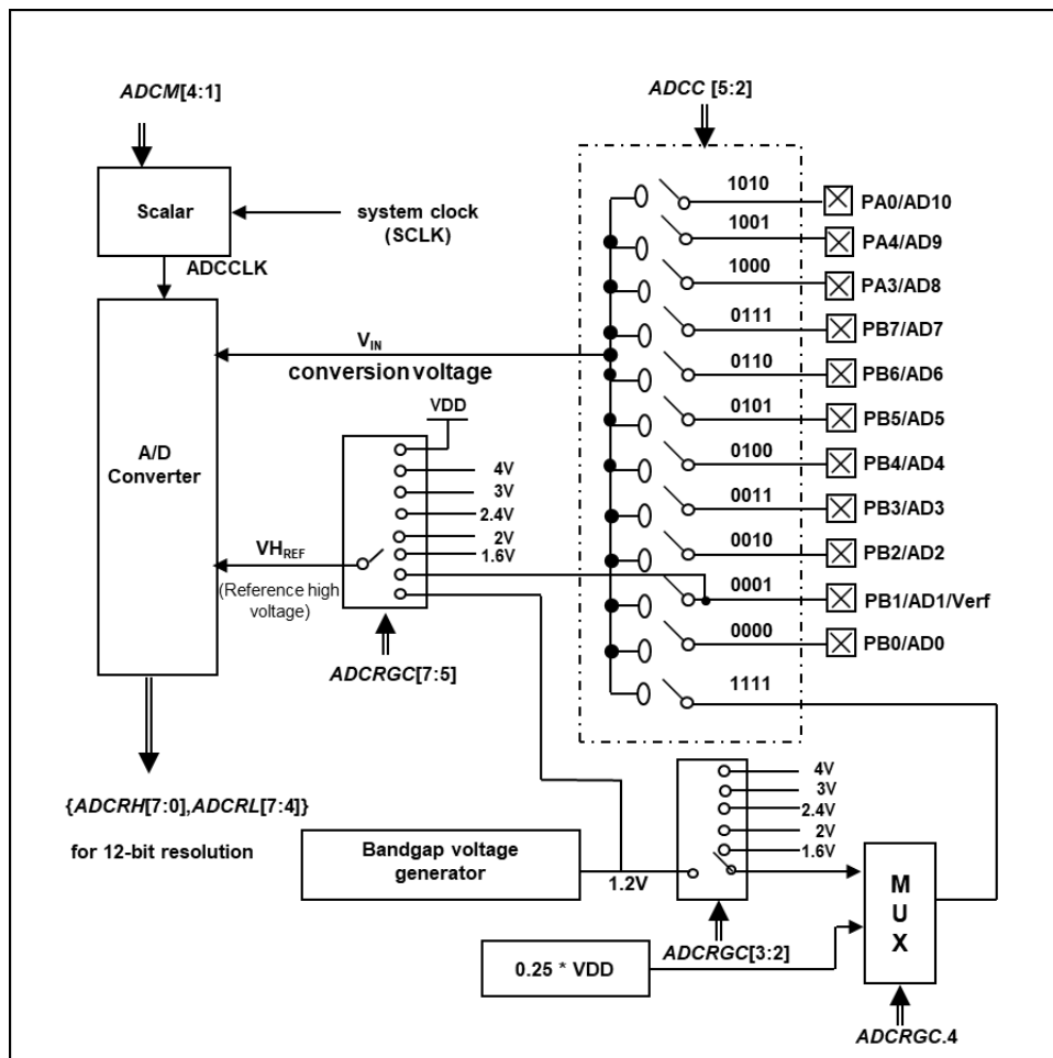
图 21: ADC 模块框图
