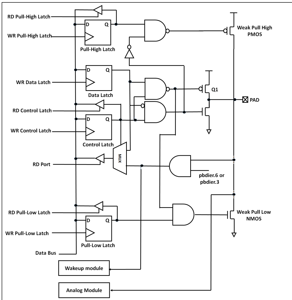
图 20: IO 引脚缓冲区硬件图
