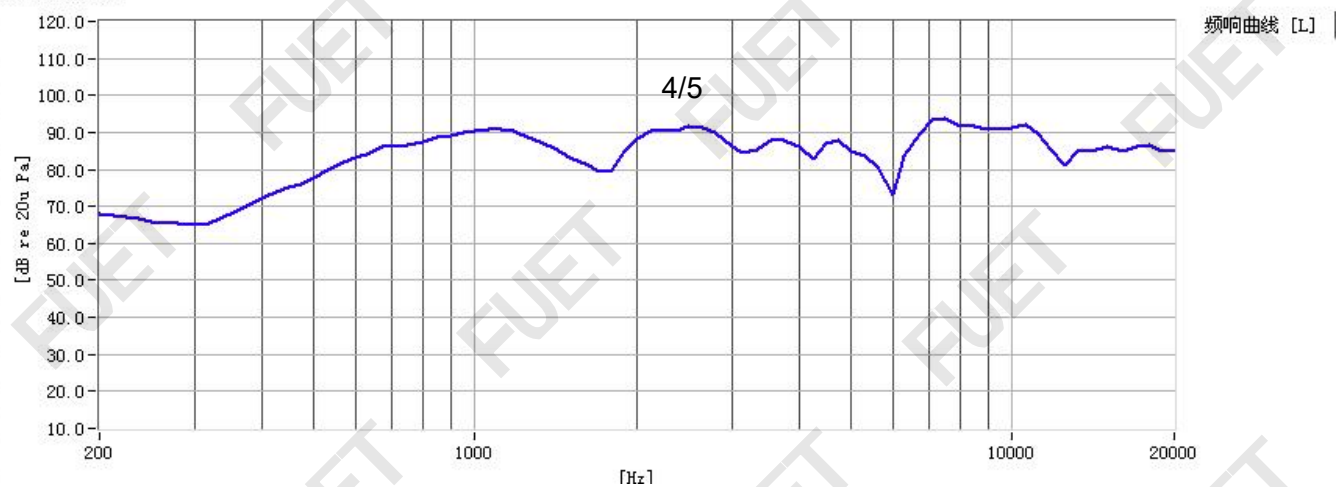
频响曲线
