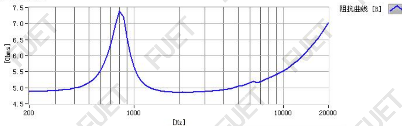
阻抗曲线
