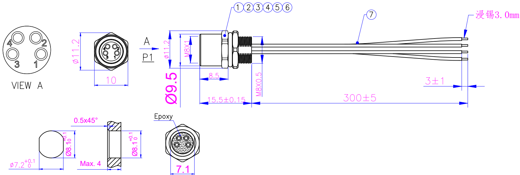
面板开孔尺寸
