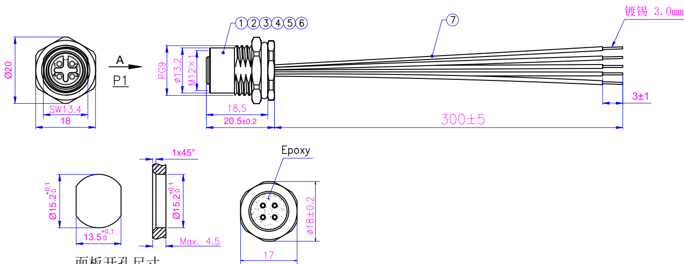
面板开孔尺寸
