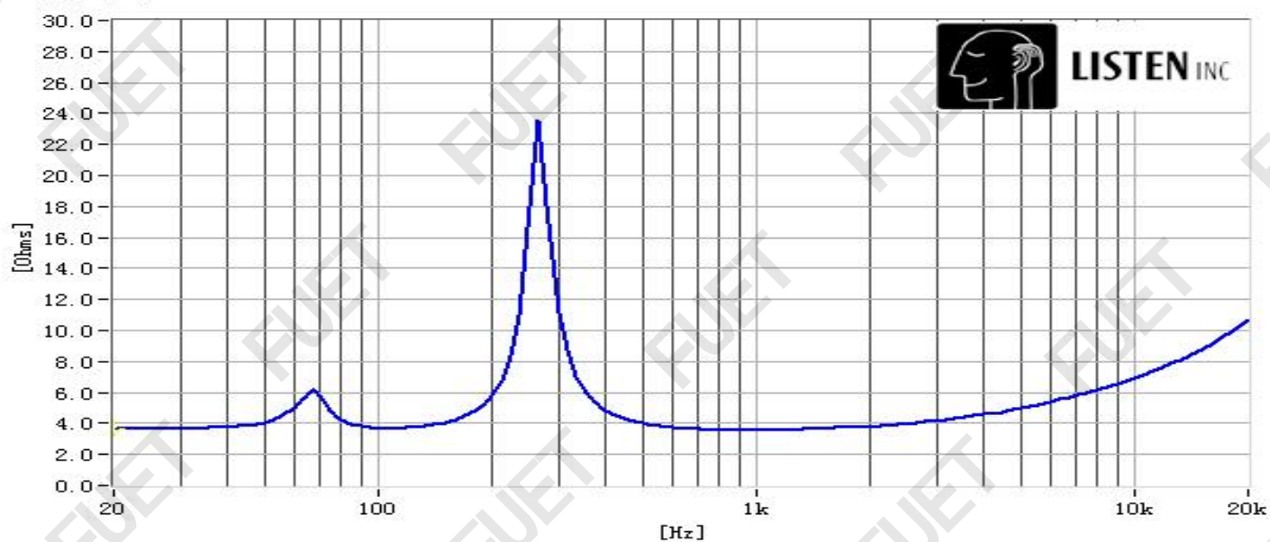
阻抗曲线
