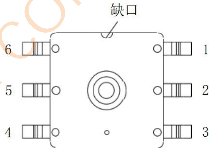
顶视图
