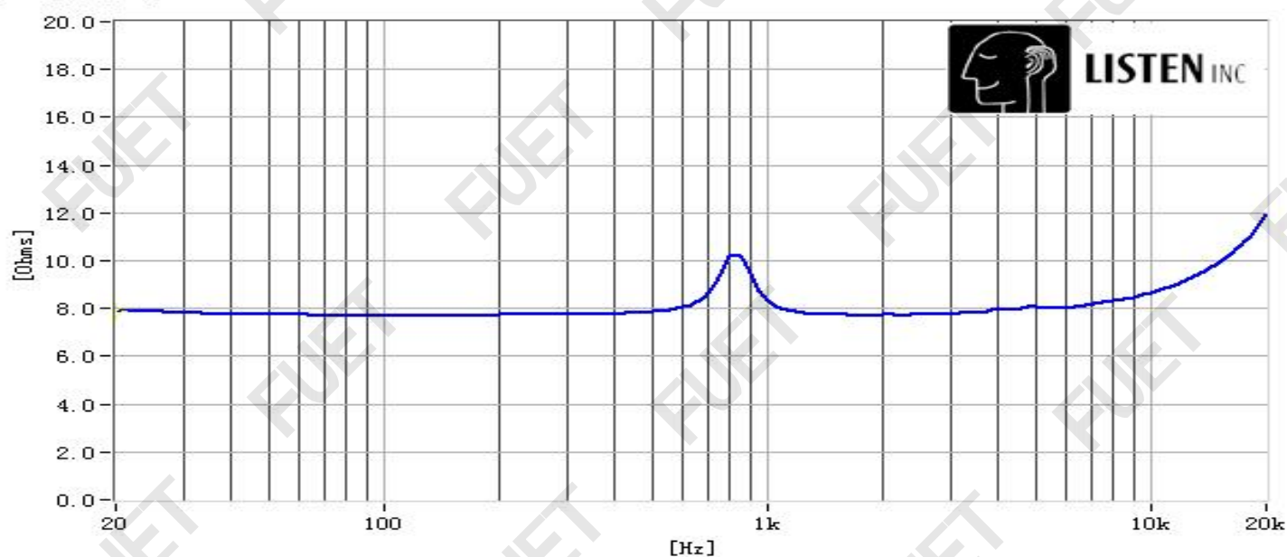
阻抗曲线
