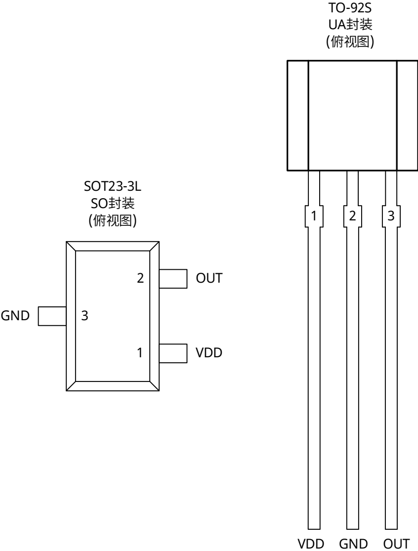
图 2 引脚定义图
