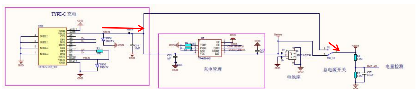
图 12 Micro USB 接口输入供电图示
