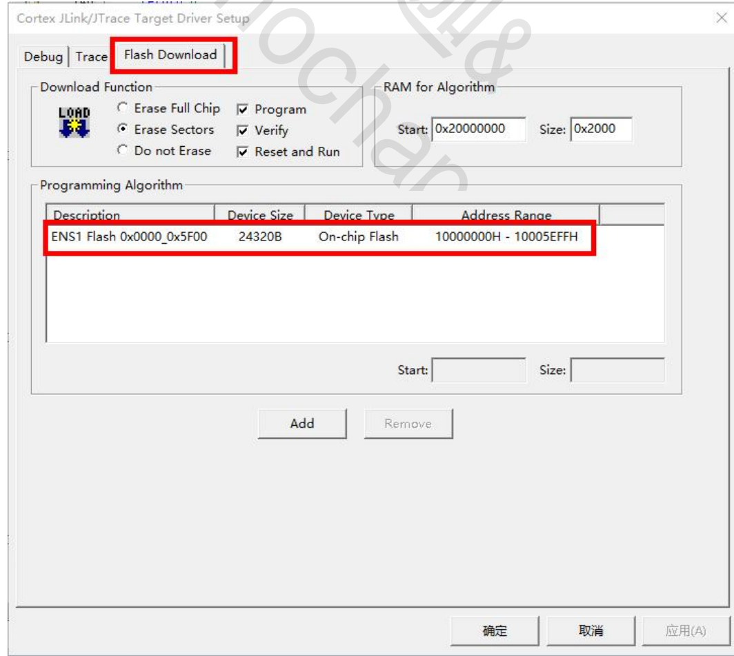
图 19 KEIL 的 flash 烧录文件选择界面
