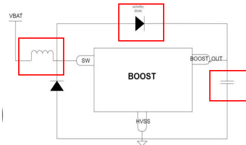
图 9 ENS001 的 BOOST 电路
