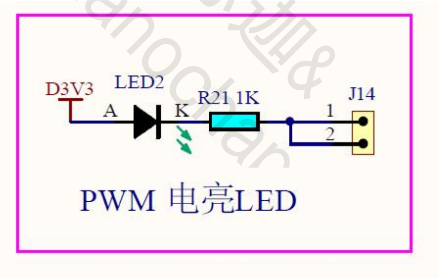
图 7 PWM 复用功能测试电路
