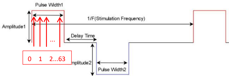
图 21 双向方波
