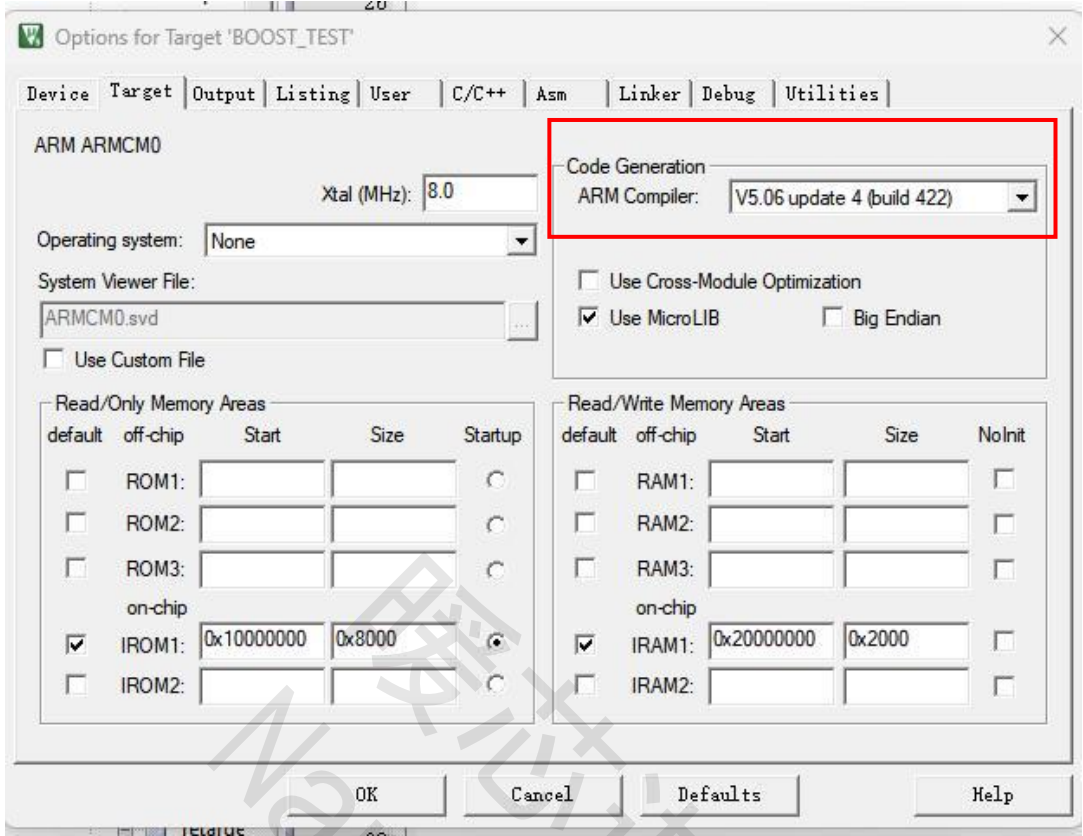
图 20 编译器选择
