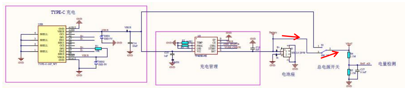
图 13 锂电池供电
