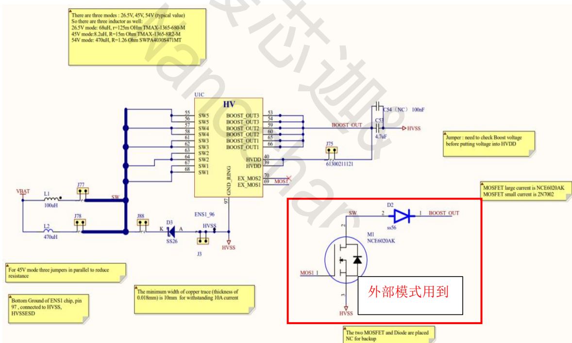
图 10 ENS001 的 BOOST 电路
