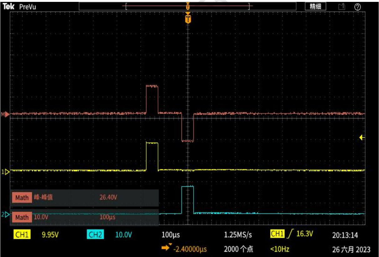
图 23 示波器处理
