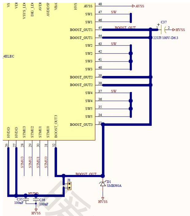
图 11 ENS001 的 boost_out 和 HVDD 引脚连接
