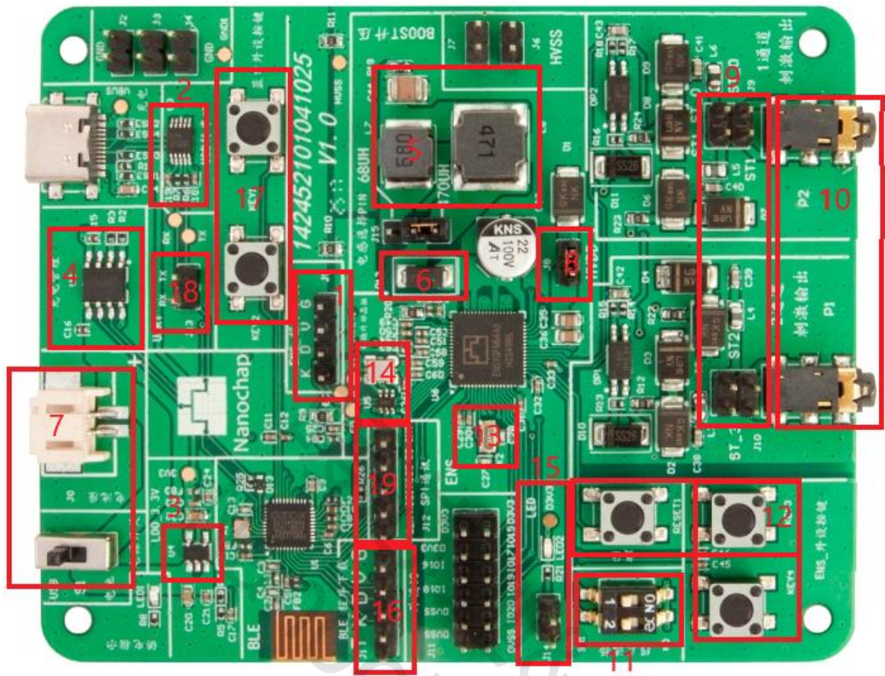
图 1 ENS1EVKG 双通道开发板图
