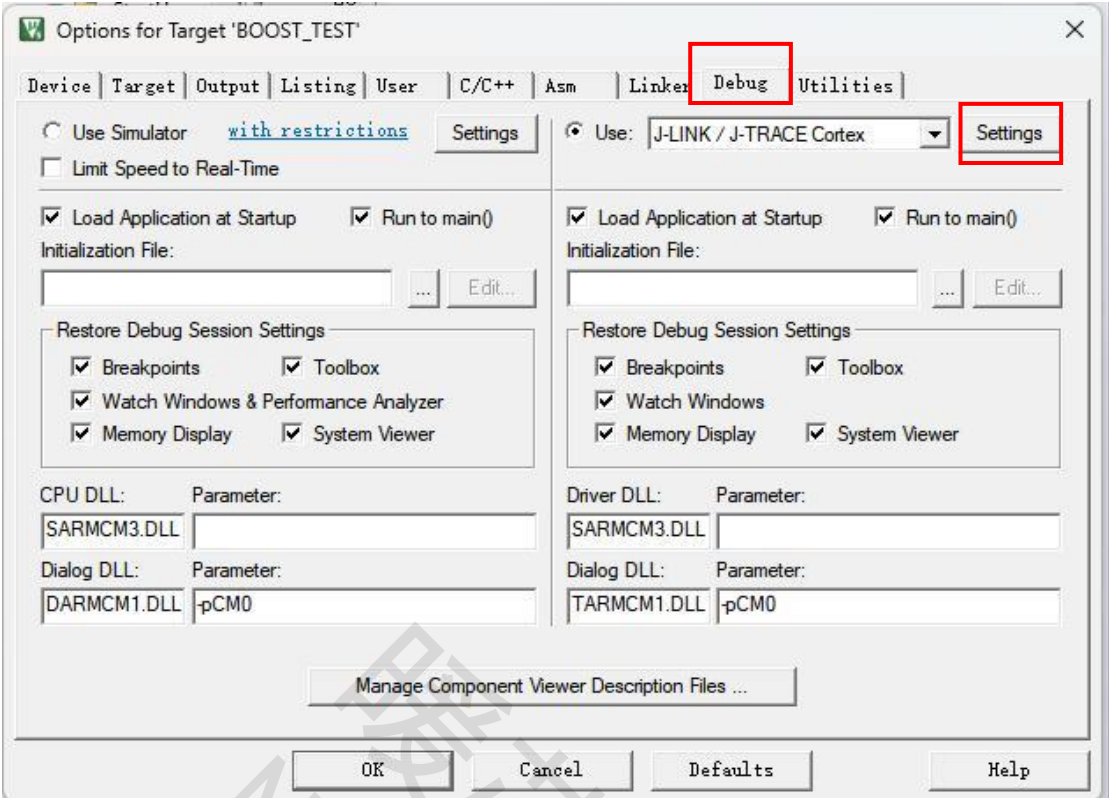
图 18 KEIL 的 options 界面
