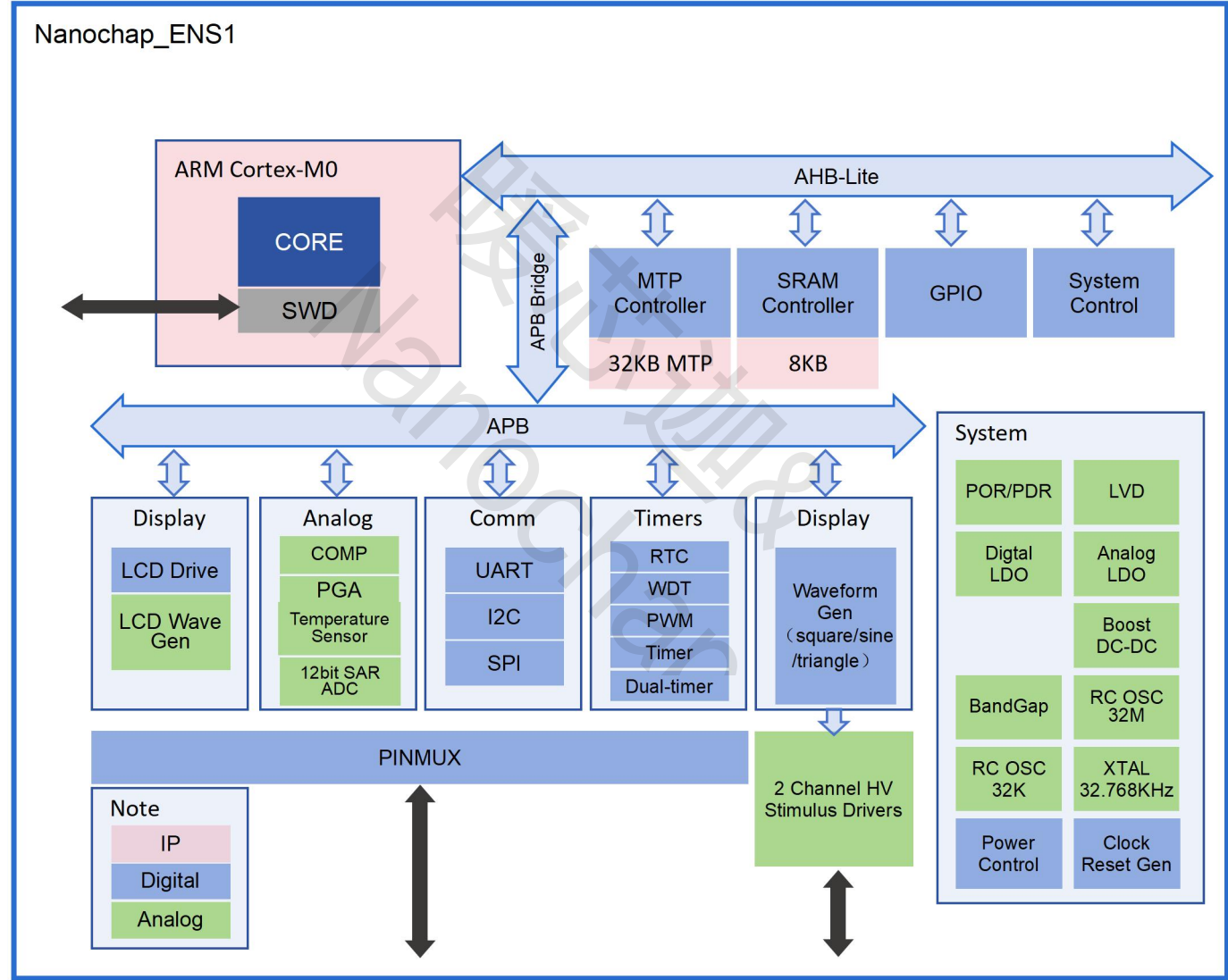
图 8 ENS001 芯片框图
