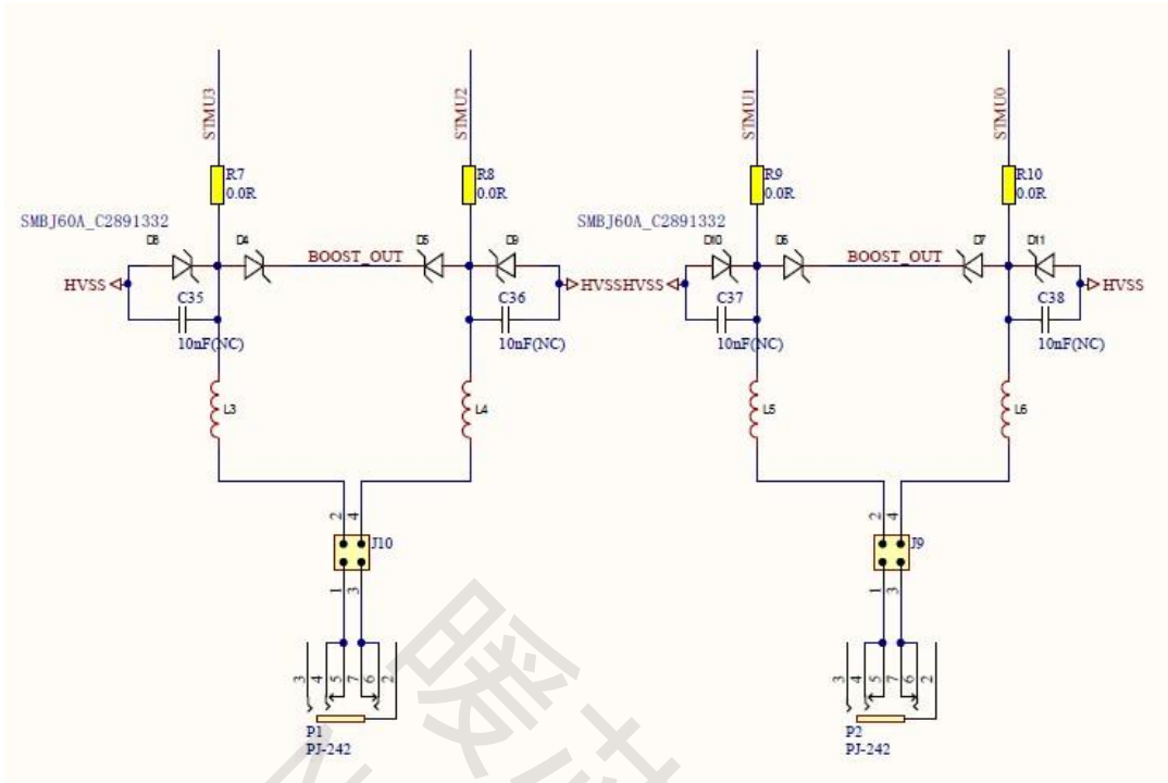
图 4 电刺激输出接口及板上测试负载
