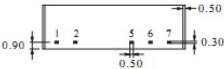
底视图
