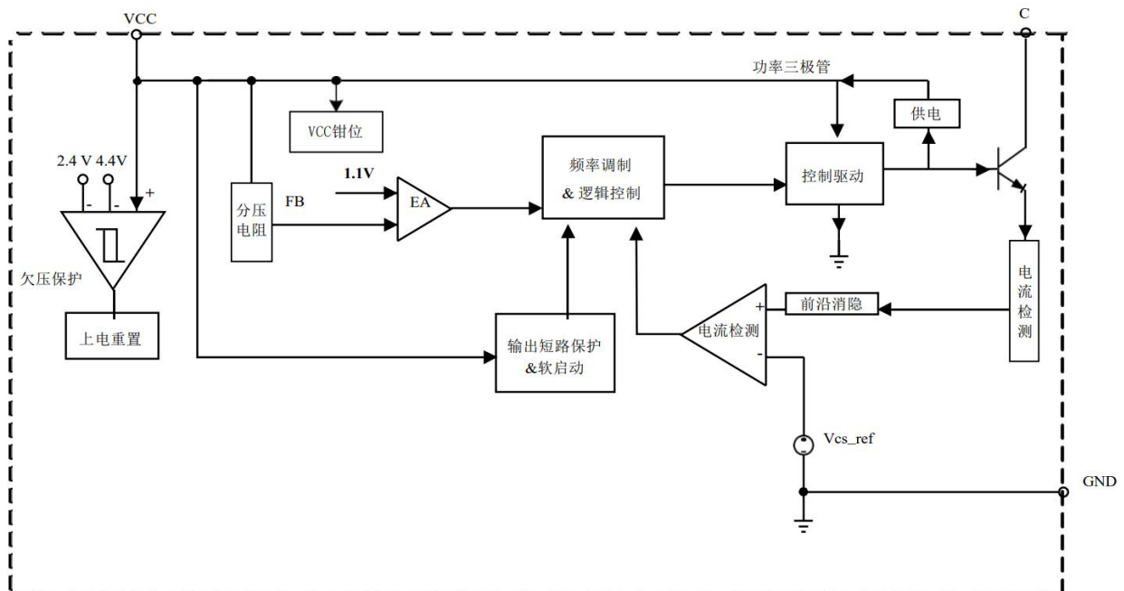
图 3. ICW4008 功能框图
