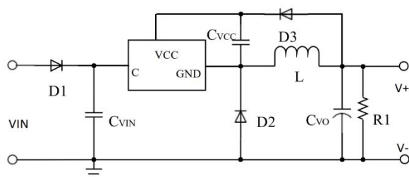
图 1. ICW4008 Buck 典型应用
