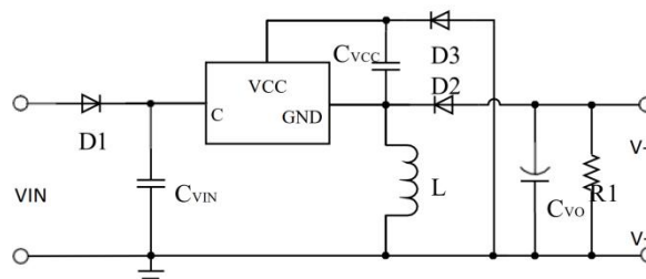
图 2. ICW4008 Buck-boost 典型应用
