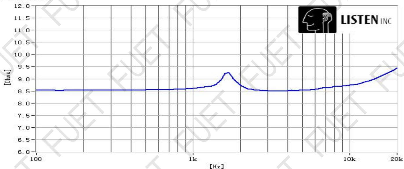
阻抗曲线
