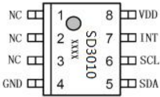
SD3010 管脚功能表
