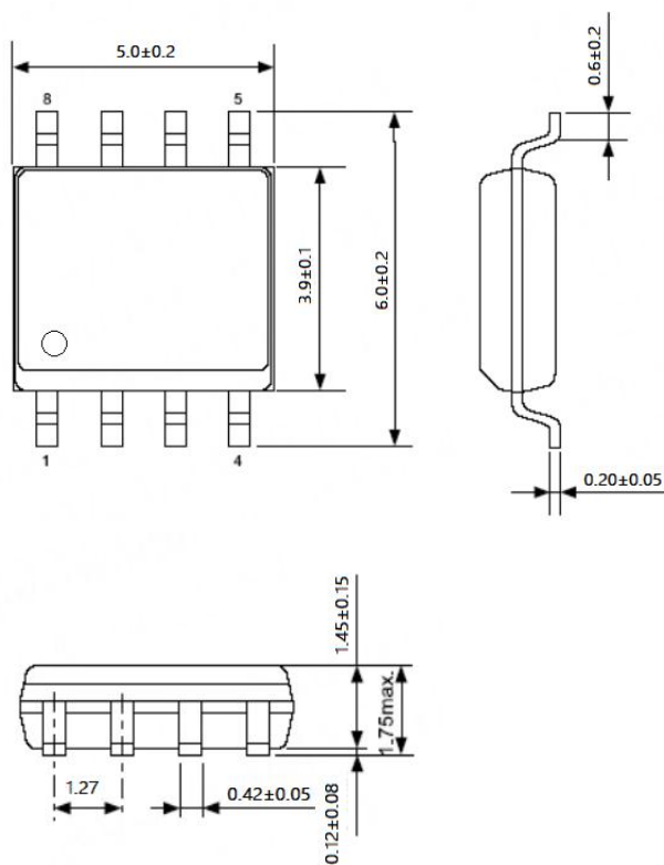
SD3010 SOP8 150mil 封装及盘装尺寸图
