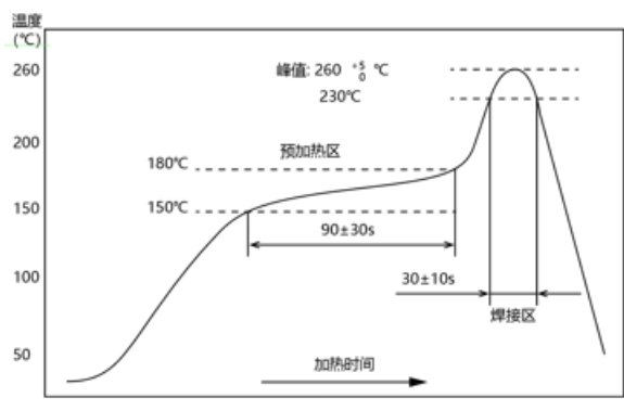
回流焊曲线图
