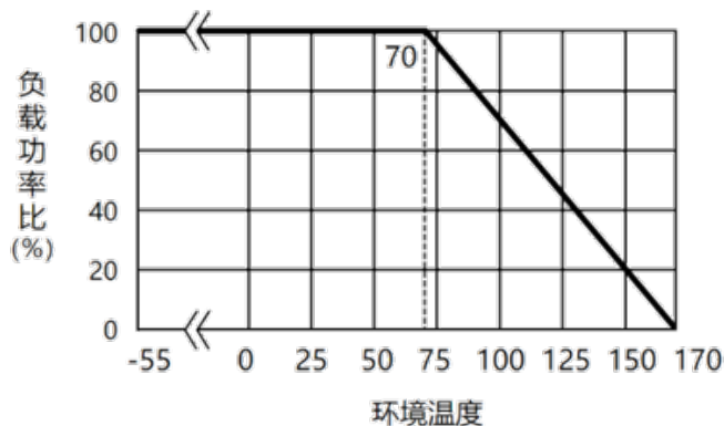
功率曲线
