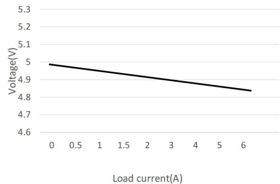
输出电流电压 (input 48V)
