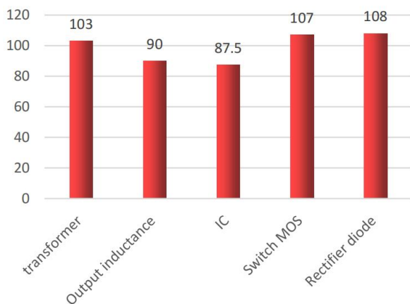
部件最高温度 条件(环境温度:27°C;输出功率: 5V / 6A; 时间: 3H)
