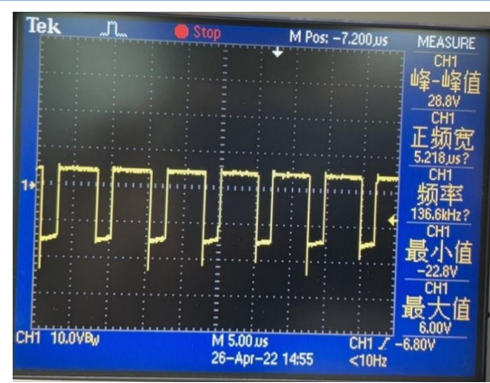
输出整流二极管
