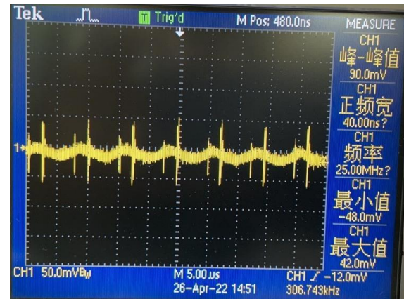
输出纹波 (5V / 6A)
