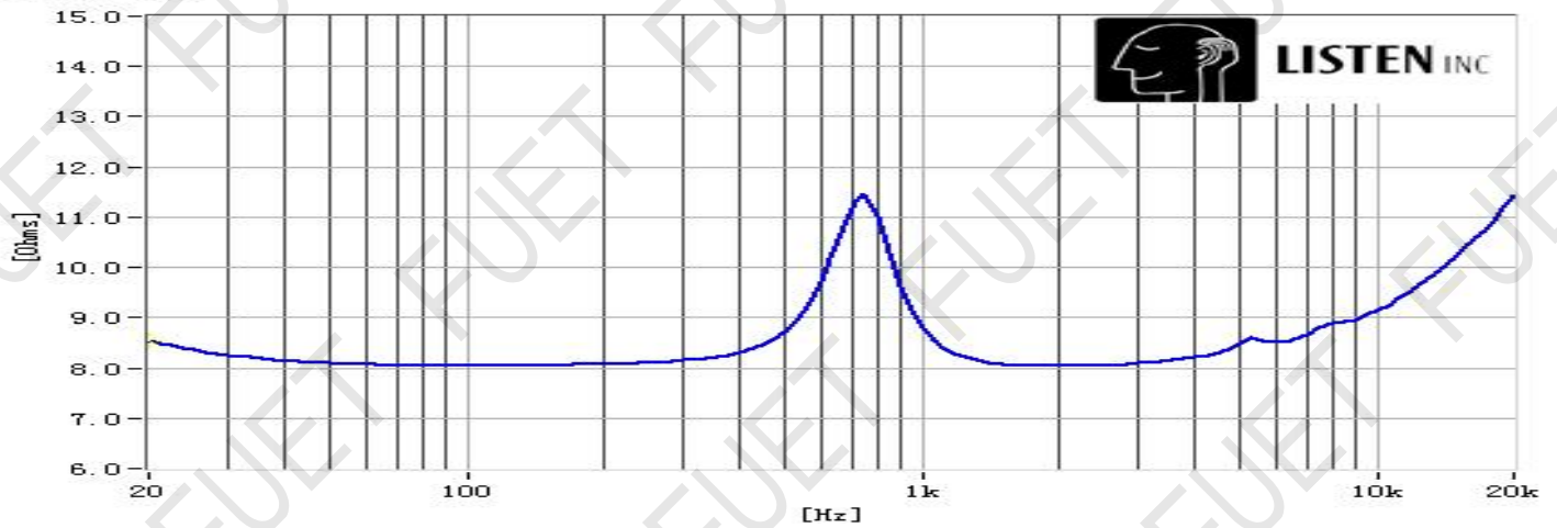
阻抗曲线
