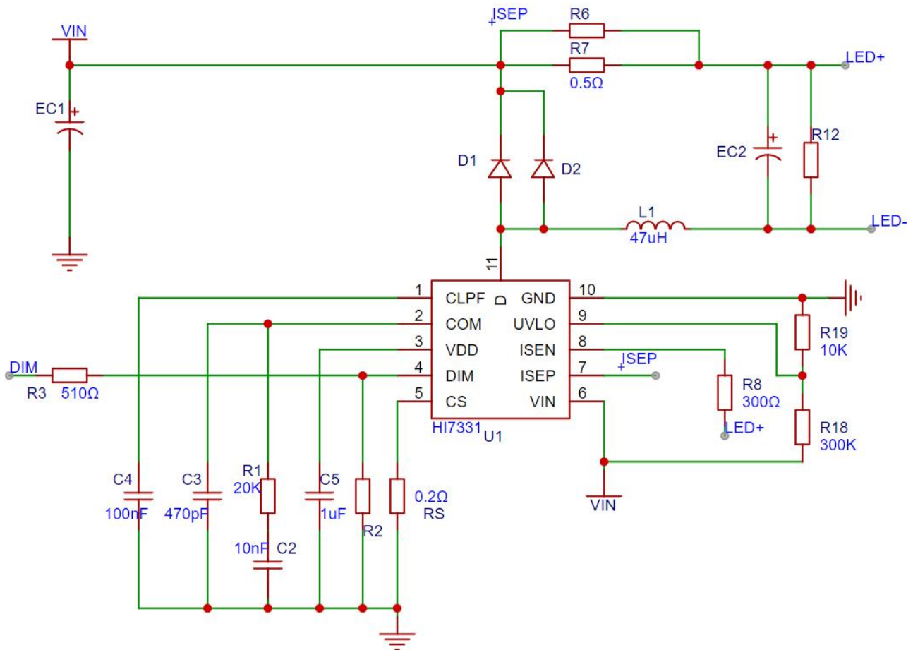
图 8.1 常规接法应用电路
