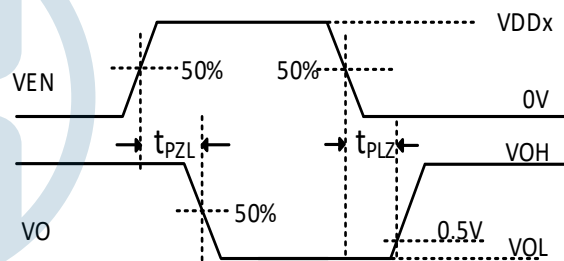
图 12. t_{pZL}/t_{pLZ} 测试波形
