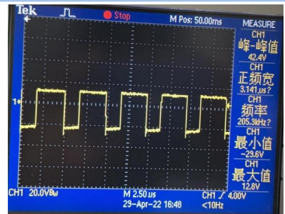
Output rectifier diode
