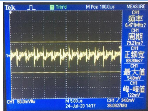
Output ripple (12V / 1.1A & 470uF)
