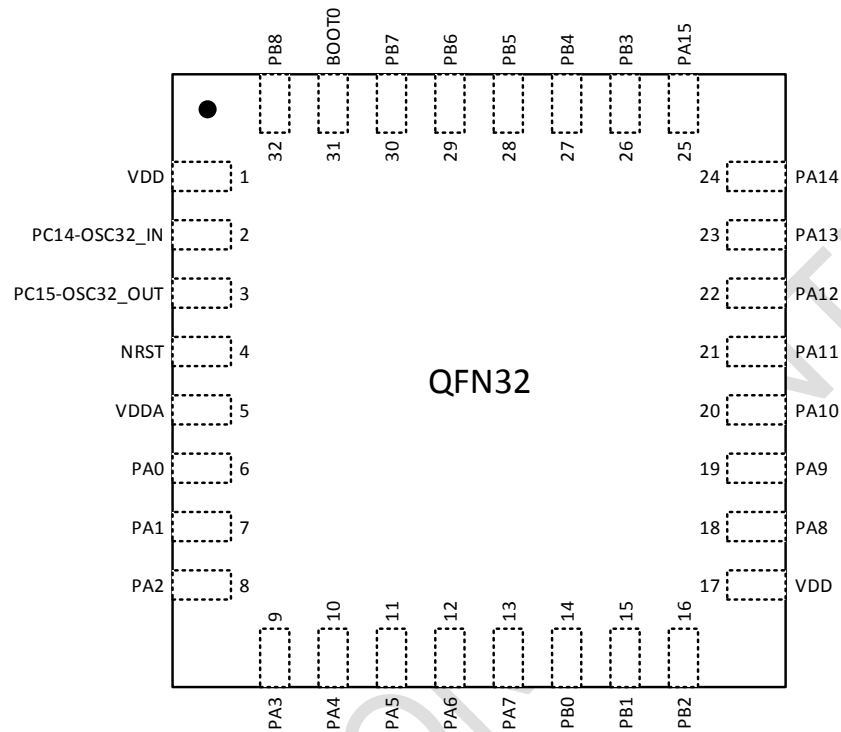
图 3-5 N32G031系列QFN32(4mx4m)引脚分布
