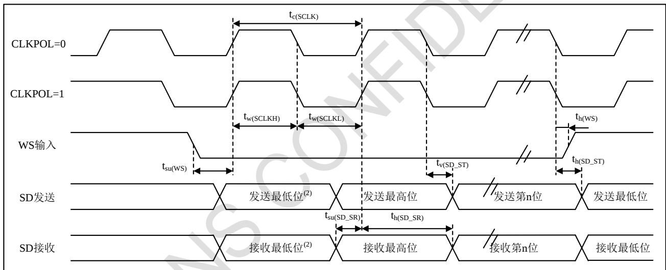
图 4-27 I 2 S从模式时序图(飞利浦协议) (1)
