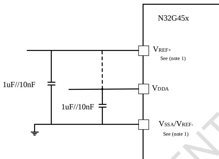
图 4-36 供电电源和参考电源去藕线路( V_{REF+} 未与 V_{DDA} 相连)
