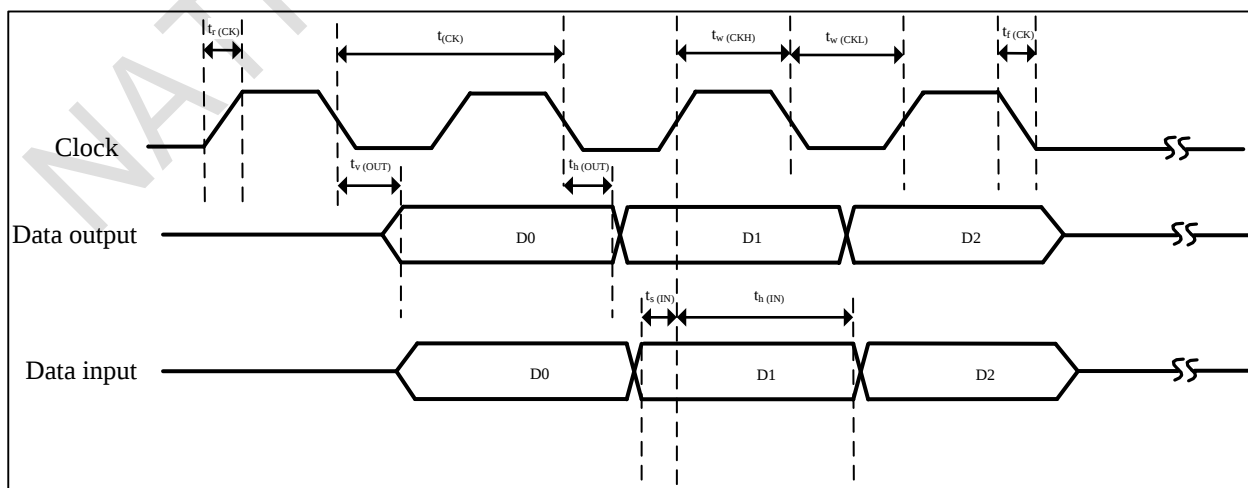
图 4-29 QSPI在SDR模式下的时序
