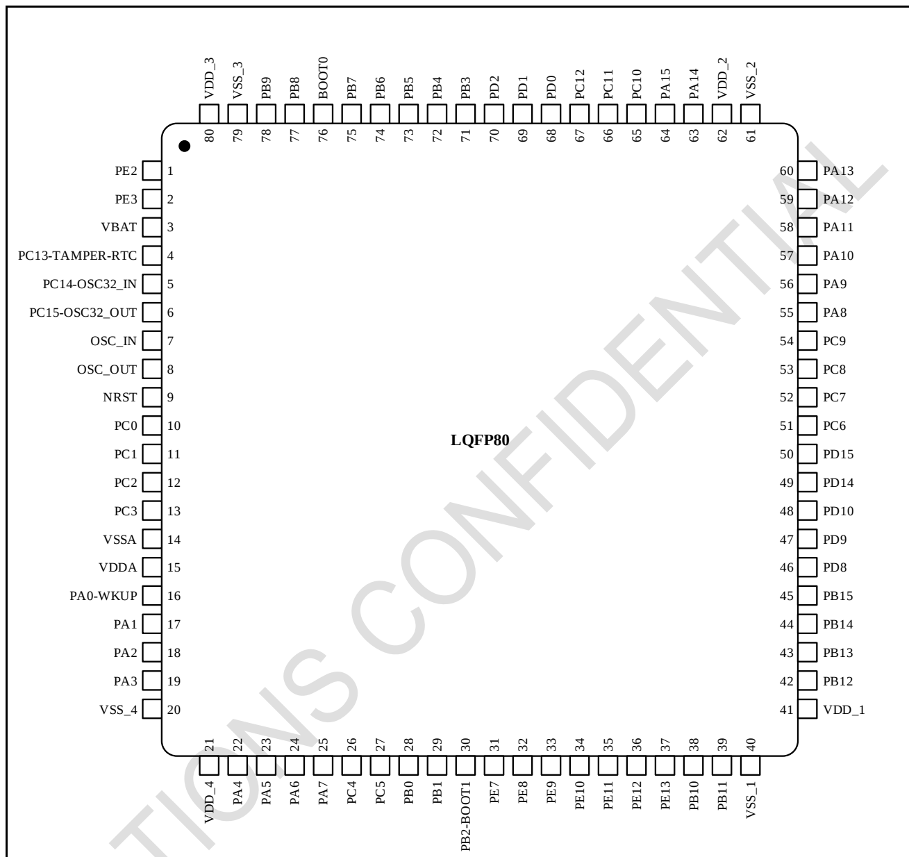
图 3-3 N32G455系列LQFP80引脚分布
