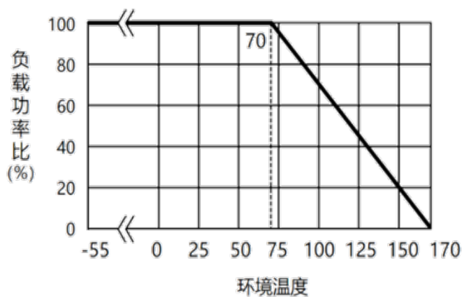
功率曲线
