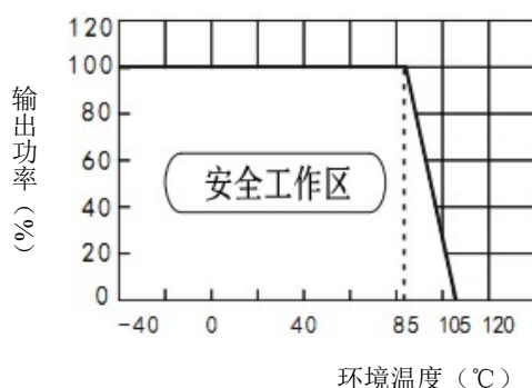
温度曲线图
