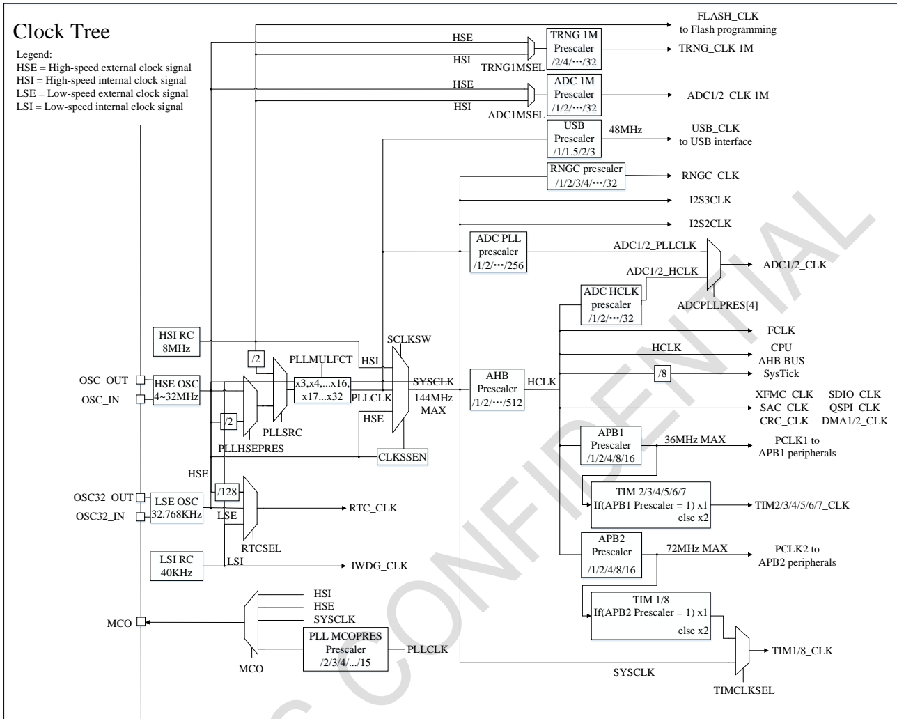
图 2-2 时钟树
