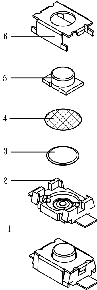
3D轴测图
