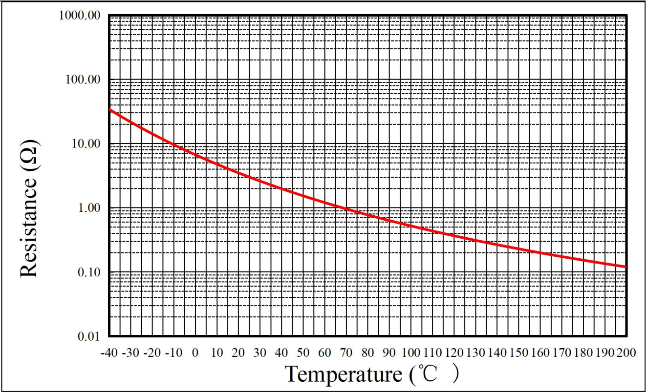
9.1.1 R-T chart 阻温特性表
