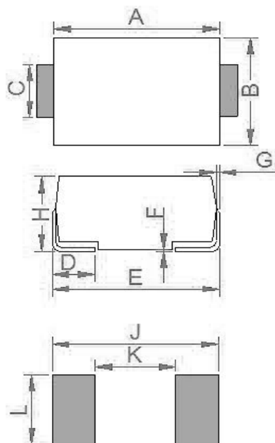
DO-214AB (SMC)
