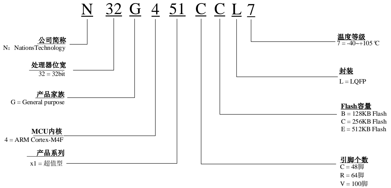
图 1-2 N32G451系列订货代码信息图示
