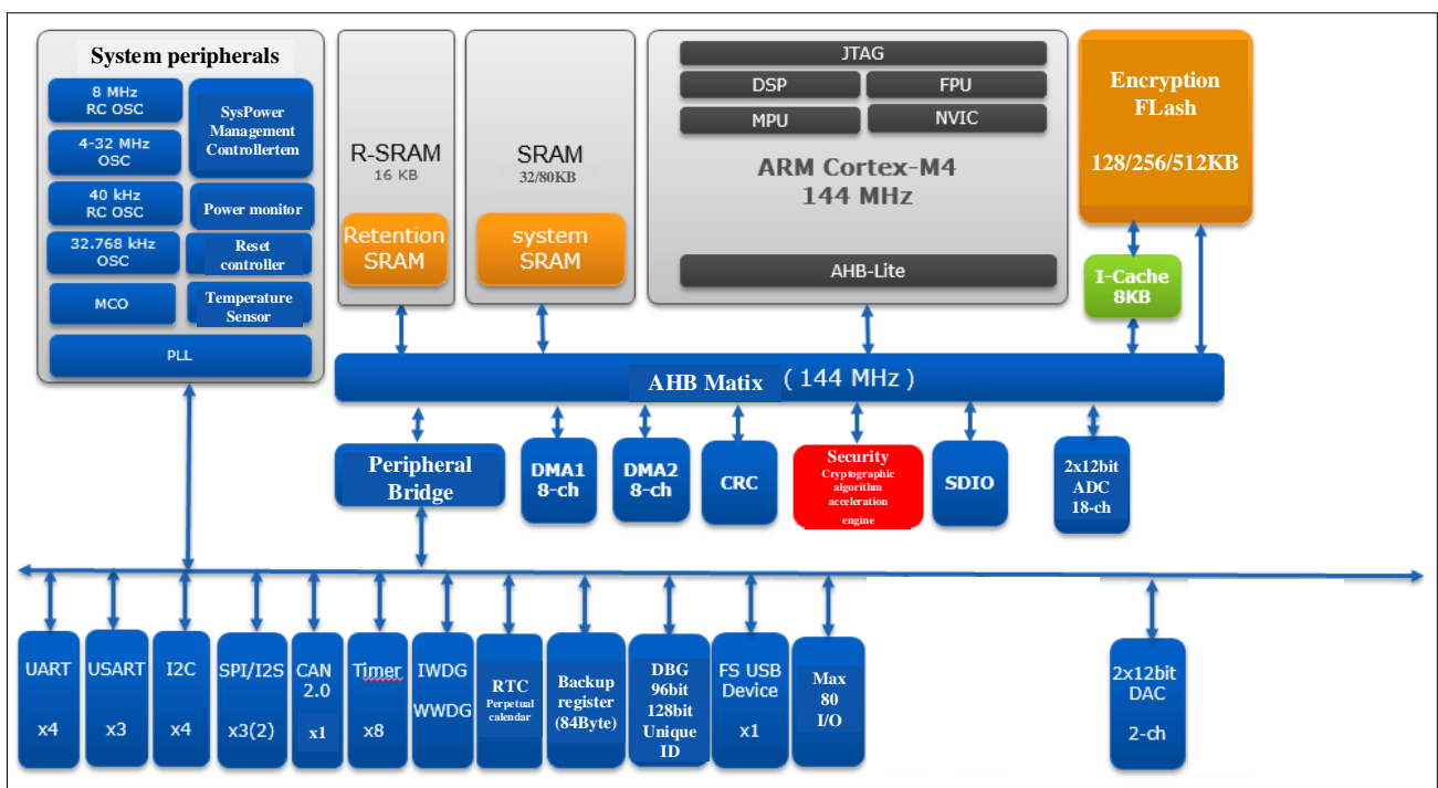
图 1-1 N32G451系列框图
