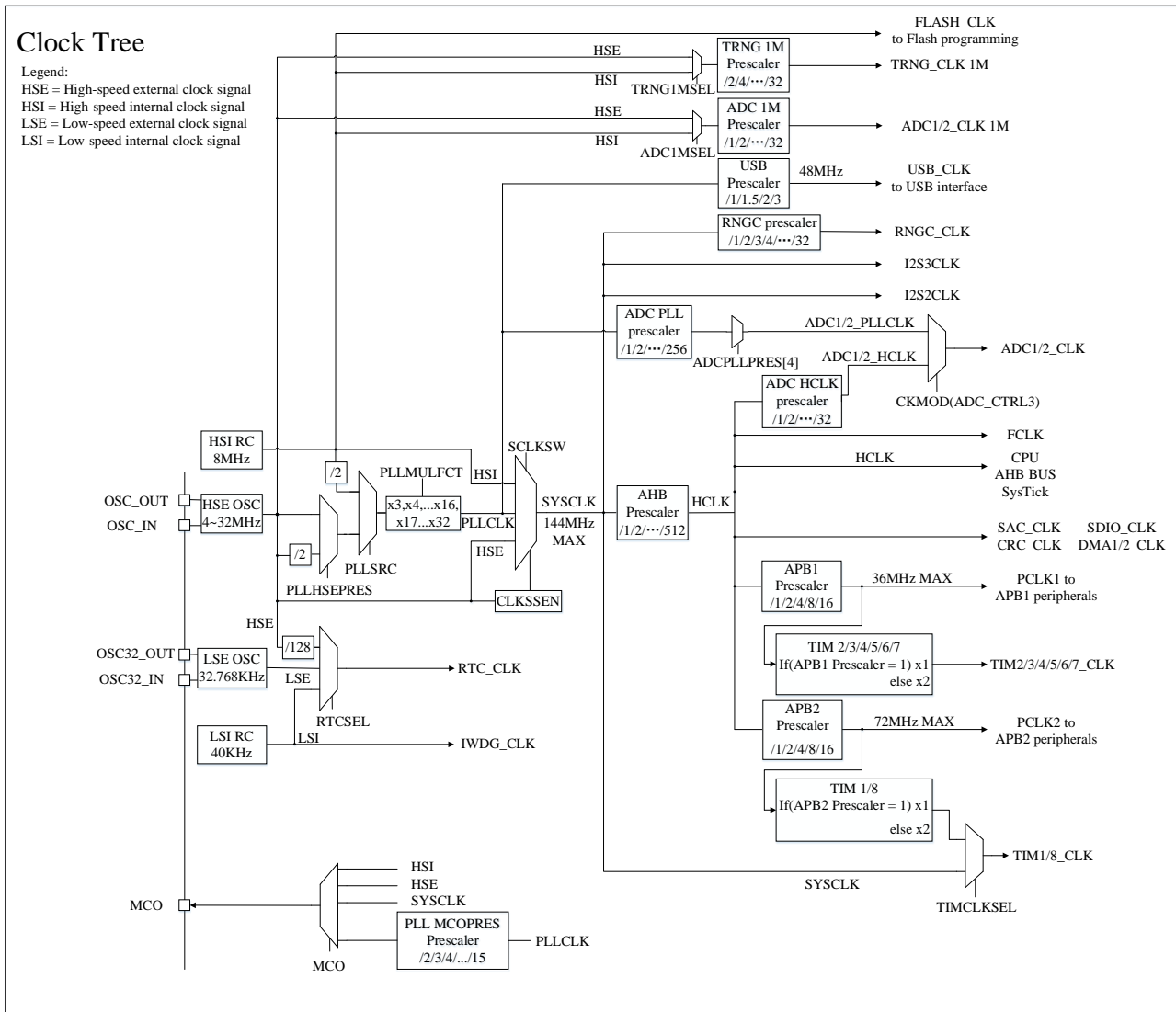
图 2-2 时钟树
