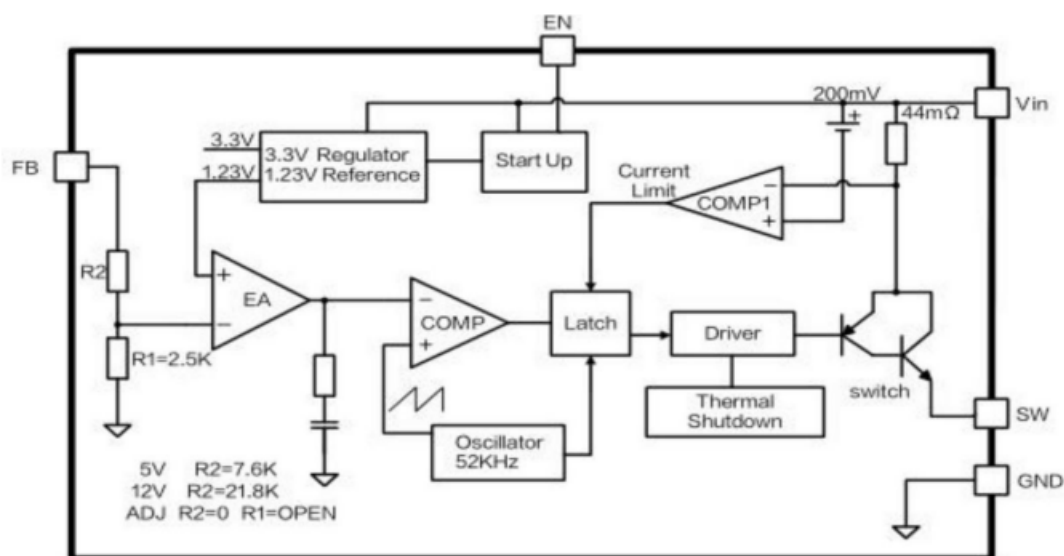
图3. 2576 方框图
