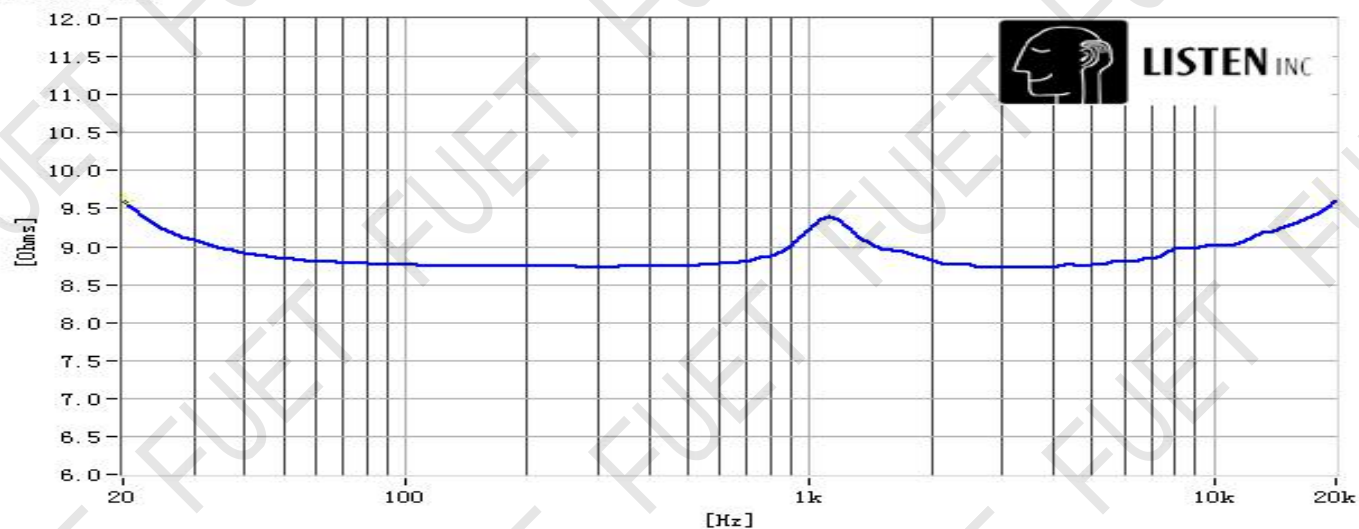
阻抗曲线
