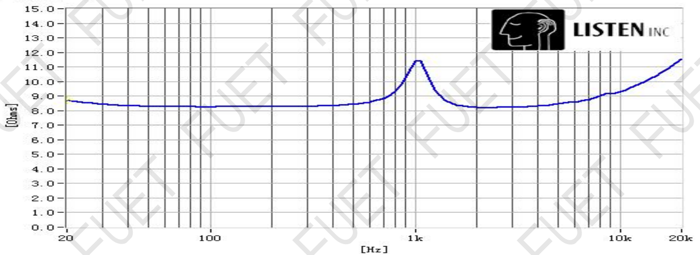
阻抗曲线
