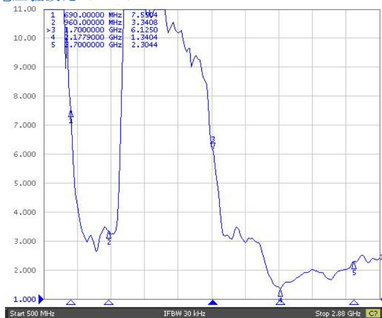
电压驻波比 (VSWR)
