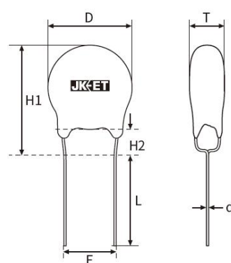
类型 D: Y 型脚
