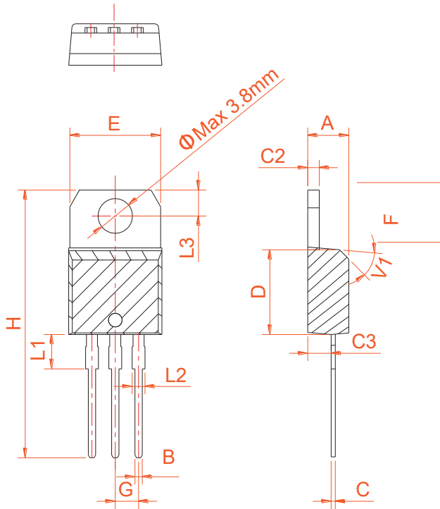
TO-220A Ins
