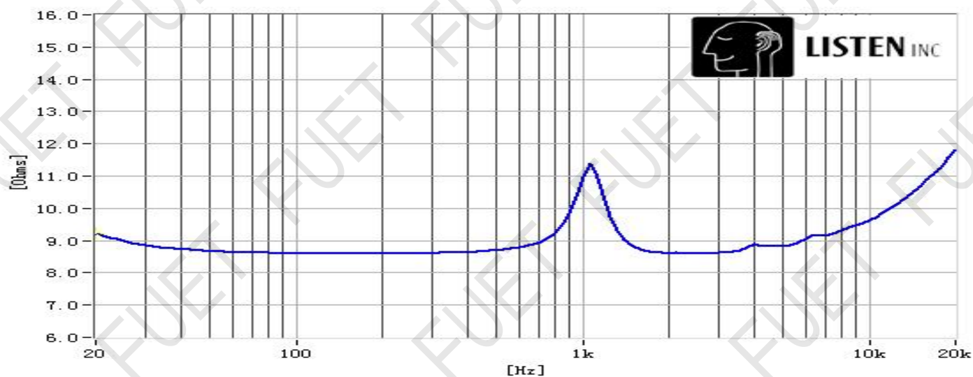
阻抗曲线
