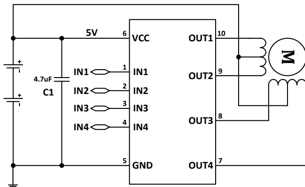
图 2、电路典型应用图
