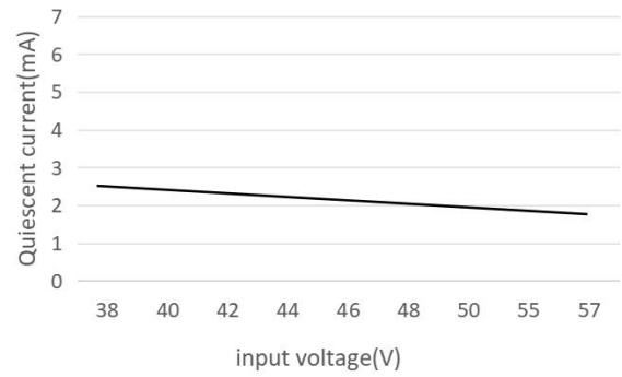
静态电流
