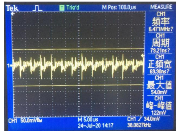
输出纹波 (12V/1.1A)
