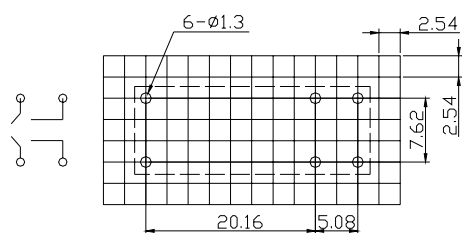
BOTTOM VIEW (2A)
