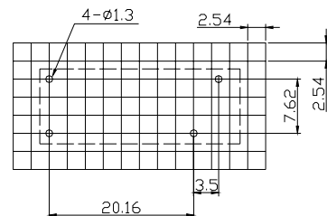
BOTTOM VIEW (1A)
