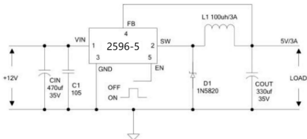
图4. 2596 系统参数测量电路(12V-5V/3A)
