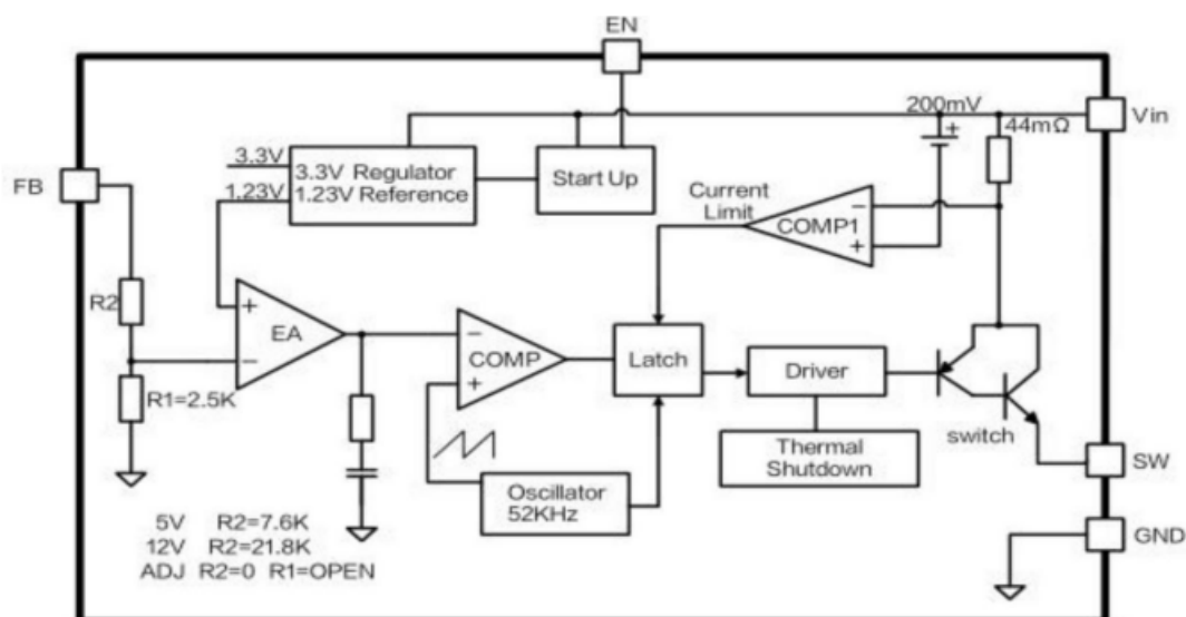
图3. 2596 方框图
